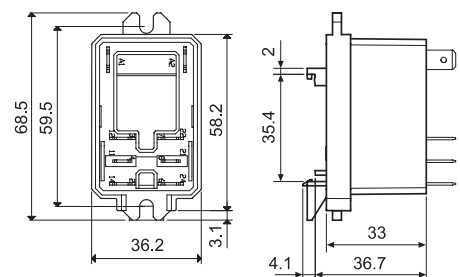
066.07 con relé
